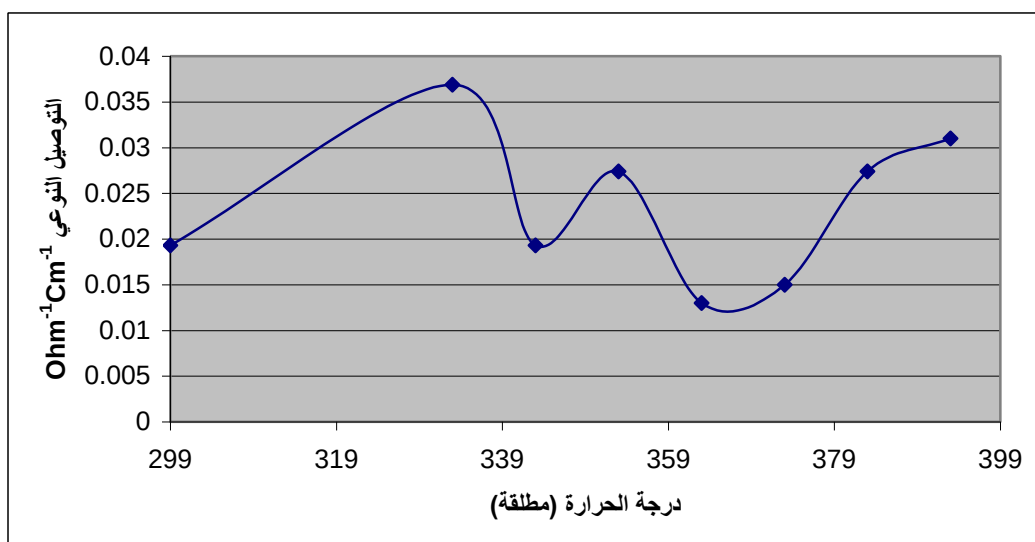
الشكل ( 9 ) العلاقة بين التوصيل النوعي ودرجة الحرارة لـ 0.02 غرام من الباراكولون سلفونيك أسد مع 0.18 غرام من البوليمر البولي أنيلين - بولي فاينيل الكحول
