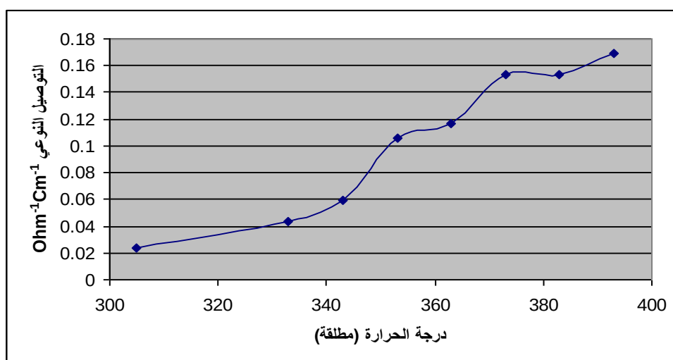
الشكل ( 10 ) العلاقة بين التوصيل النوعي ودرجة الحرارة
