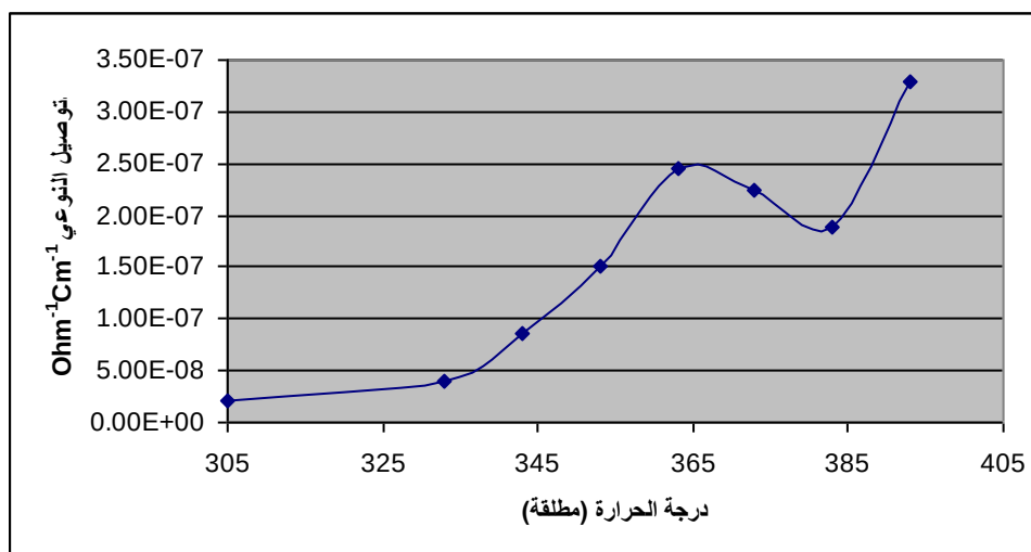
الشكل ( 8 ) العلاقة بين قيم التوصيل النوعي ( \kappa ) ودرجة الحرارة لنموذج البولي أنيلين - بولي فاينيل الكحول بدون تشويب بمادة الباريتولوين سلفونيك أسد PTSA
