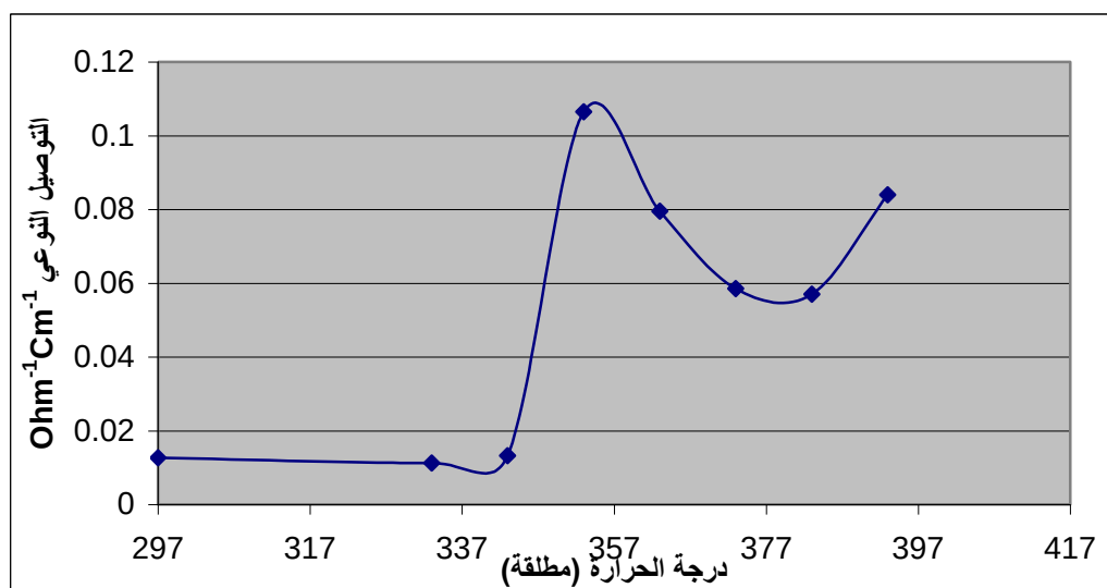
الشكل ( 12 ) العلاقة بين التوصيل النوعي ودرجة الحرارة لـ 0.08 غرام من الباراكولون سلفونيك أسد مع 0.12 غرام من البوليمر البولي أنيلين - بولي فاينيل
